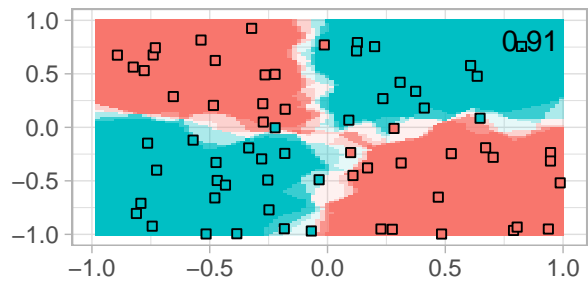
kkn
