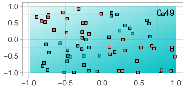
lin. svm
